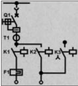
Arranque estrella-triángulo
