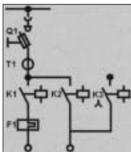
Arranque estrella-triángulo
