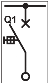
Interruptor automático como entrada/salida fijo
