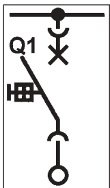
Interruptor automático como entrada/salida extraíble
