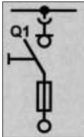
Interrupor-fusibles
