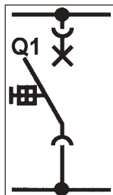
Interruptor automático como acoplamiento de barras extraíble.
