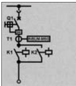
Arranque directo dos sentidos de giro, con INSUM®
