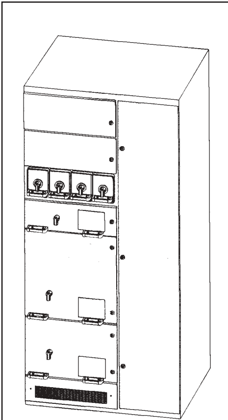
Columna para unidades extraíbles con compartimentos para aparatos, barras y cables.
